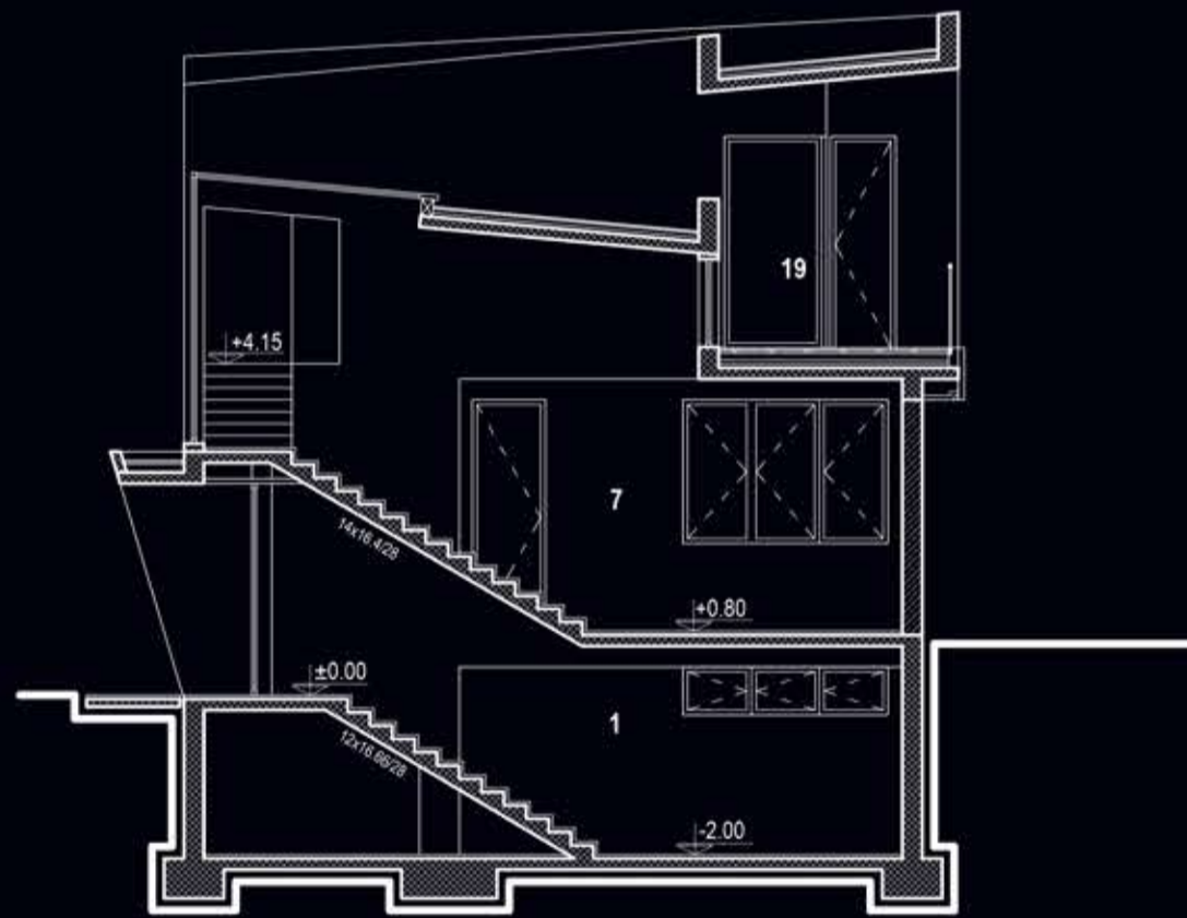
Разрез 1-1 SECTION 1-1
