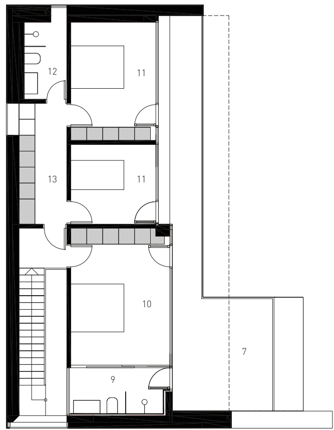
floor plan level 3/ план ниво 3
