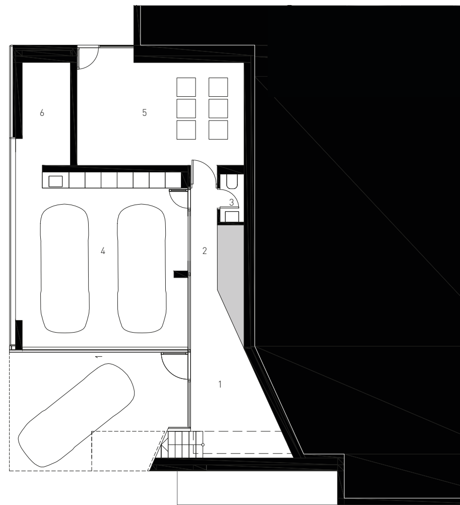
floor plan level 1/ план ниво 1
