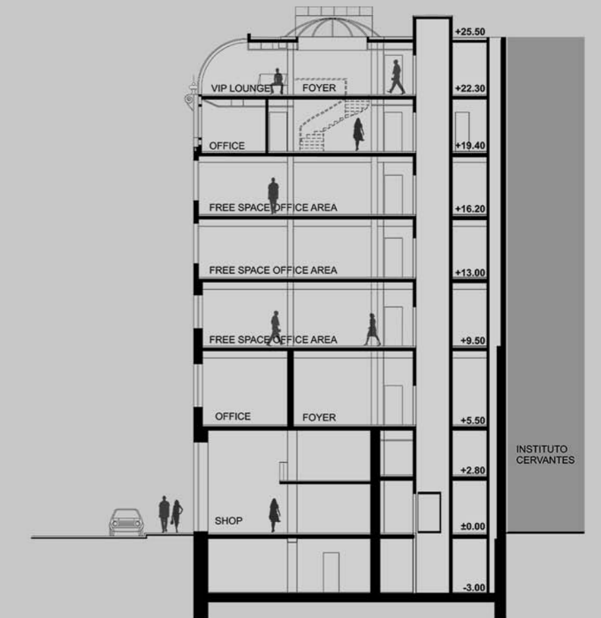
разрез вариант 1
