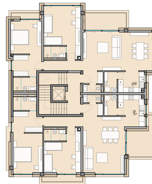
РАЗПРЕДЕЛЕНИЕ ЕТАЖ 3
