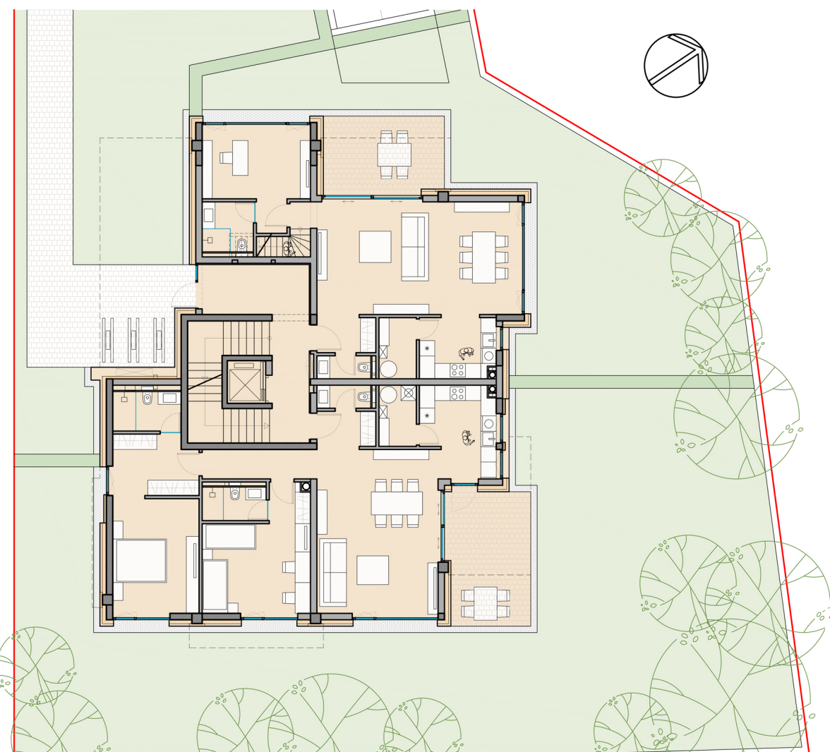
РАЗПРЕДЕЛЕНИЕ ЕТАЖ 1
